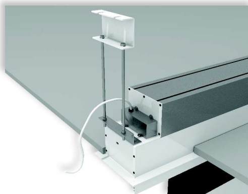
VUE COTÉ GAUCHE (MOTEUR)
