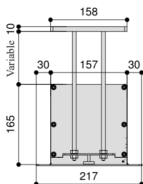
CAISSON VUE DE COTE
