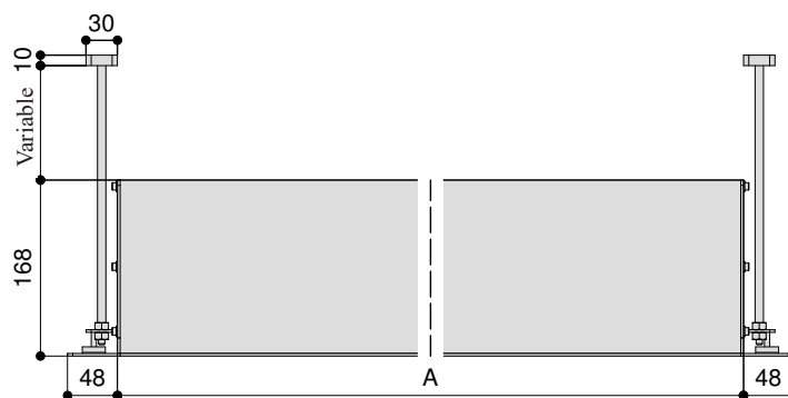
CAISSON VUE DE FACE
