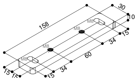
DIMENSIONS AU PLAFOND
